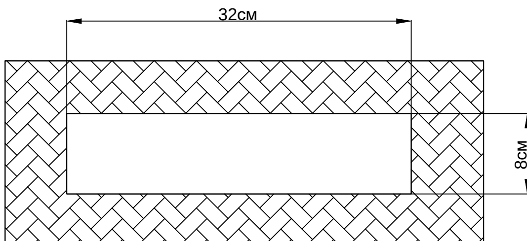
130. Размер отверстия под плитку
