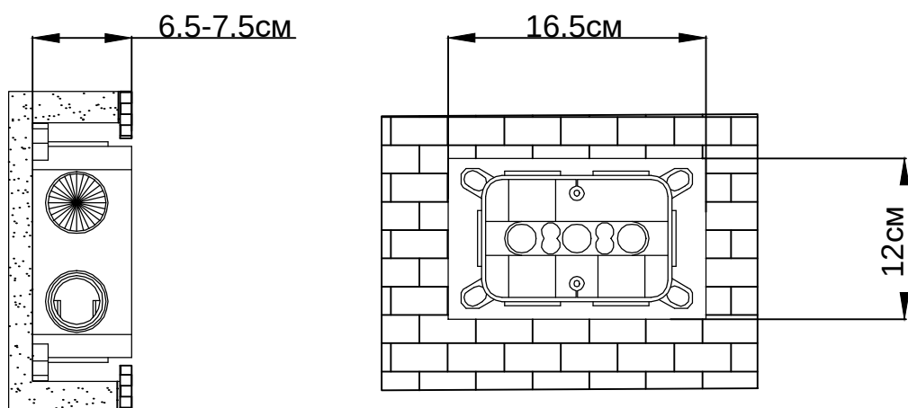
Скрытый корпус — блок управления душем
