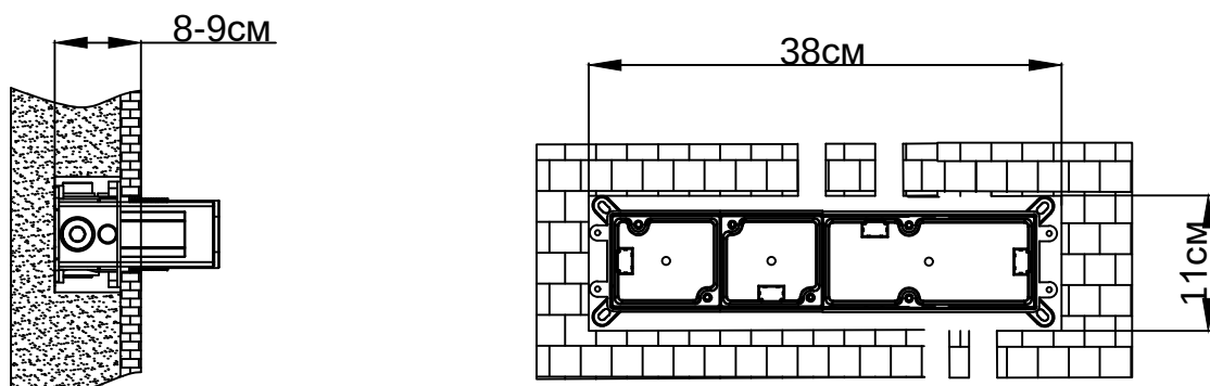
130. Скрытый корпус смесителя
